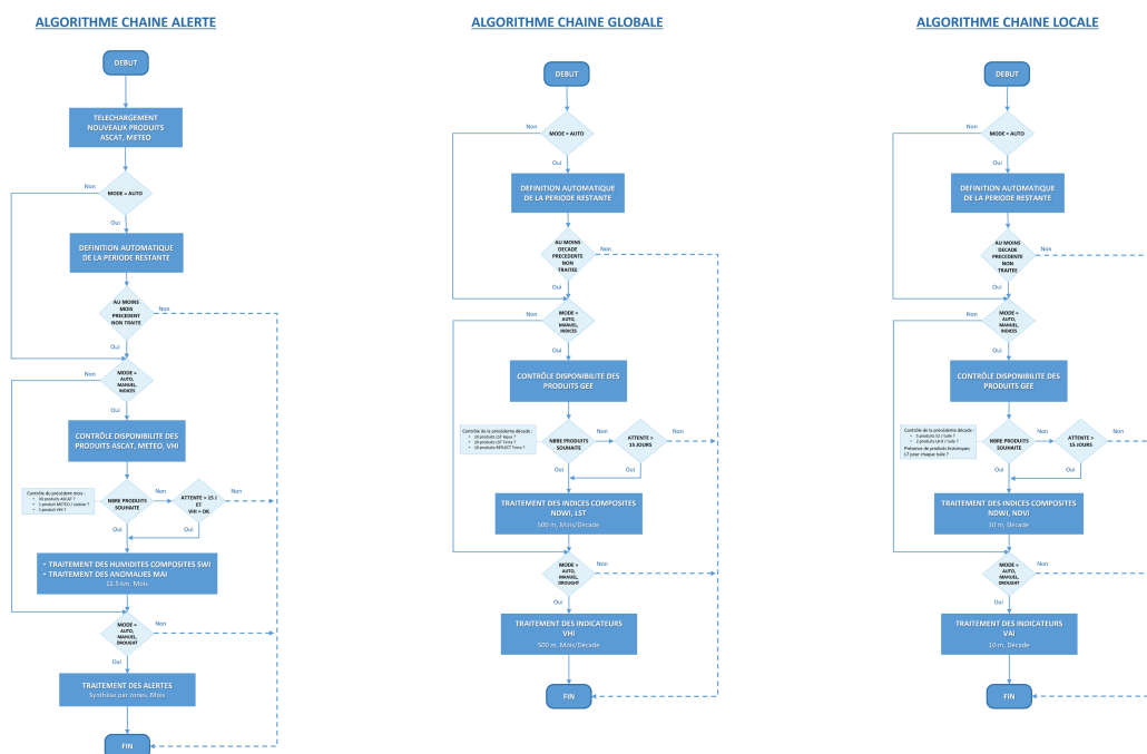
Figure 4: Description du fonctionnement détaillée des chaînes
