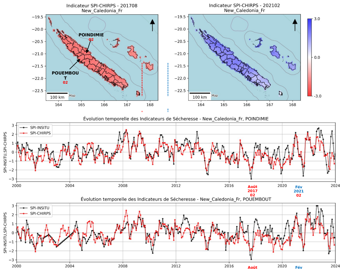
Figure : Cartes sur la Nouvelle-Calédonie de l'indicateur de sécheresse météorologique SPI-3 mois calculé à partir des données CHIRPS, pour les mois d'août 2017 et février 2021. Les séries temporelles correspondent aux données SPI-CHIRPS et SPI-INSITU (stations Météo-France) agrégées sur deux communes : Poindimié (côte Est) et Pouébo (côte Ouest).
