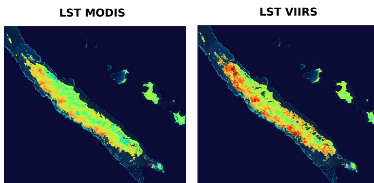
Figure : Températures LST 2019_11_D2
