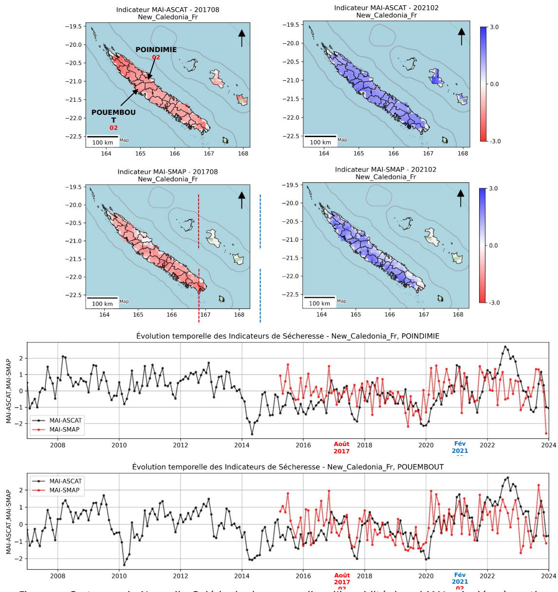
Figure : Cartes sur la Nouvelle-Calédonie des anomalies d'humidité du sol MAI calculées à partir des données ASCAT puis SMAP, pour les mois d'août 2017 et février 2021. Les séries temporelles correspondent aux données agrégées sur deux communes : Poindimié (côte Est) et Pouembout (côte Ouest).
