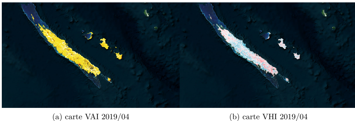
Figure 7: Comparaison des cartes VAI et VHI pour le mois d'avril 2019
