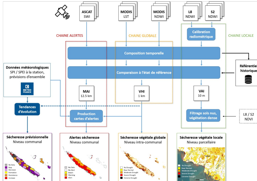
Figure Chaîne de production de l'indicateur sécheresse
