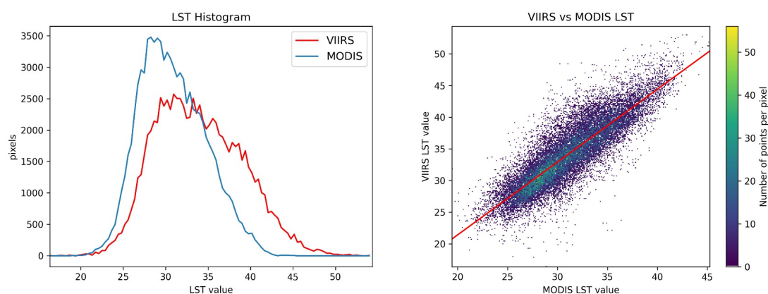
Figure : Comparaison d'histogrammes et modélisation linéaire pour les températures LST VIIRS vs LST MODIS ("chaîne"), le 2019_11_D2 sur la Nouvelle-Calédonie.
