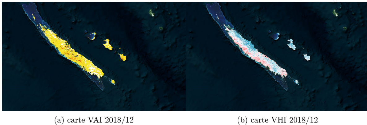
Figure 6: Comparaison des cartes VAI et VHI pour le mois de décembre 2018
