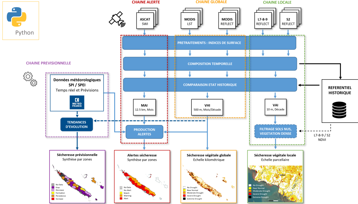
Figure 3: Le système de suivi et la prévision de la sécheresse dans les territoires du Pacifique
