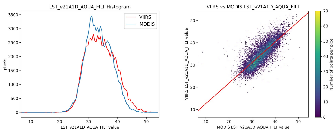
Figure 3 : Comparaison d'histogrammes et modélisation linéaire pour les températures LST VIIRS vs LST MODIS ("à tester"), le 2019_11_D2 sur la Nouvelle-Calédonie.
